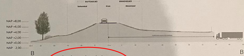
Profiel BB' Constructie stabiliteit
