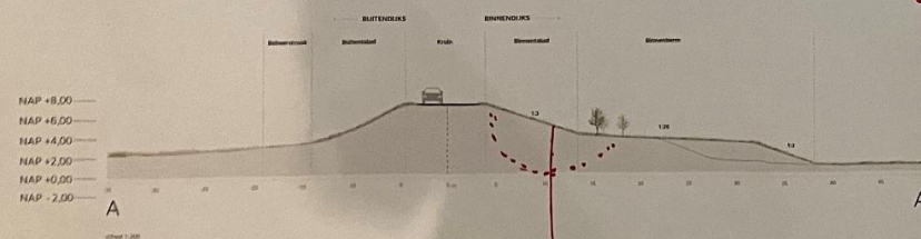
Profiel AA' Verbreding binnenberm
