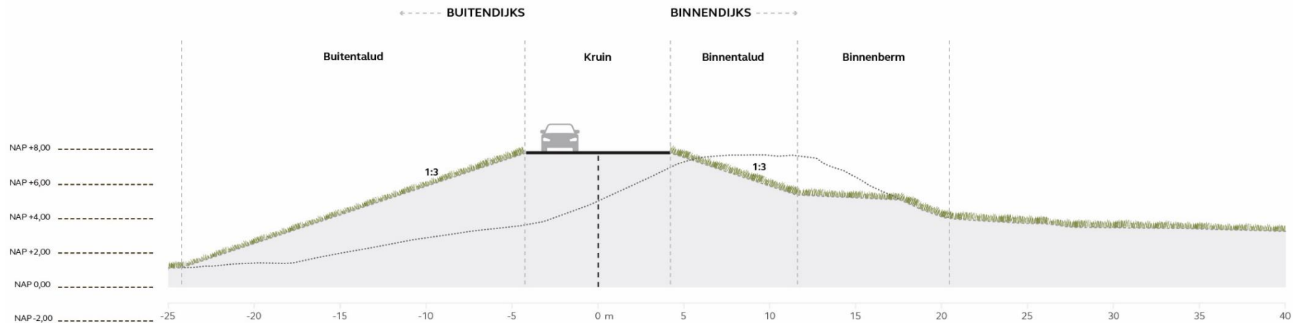
Dijkvak 26a Buitenwaartse asverschuiving (alternatief 2)
