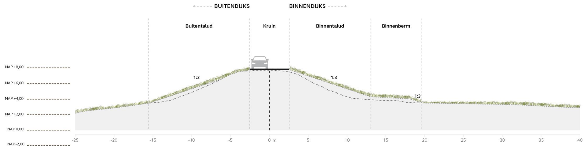
Dijkvak 25b Kruinverhoging en binnenberm (alternatief 1)
