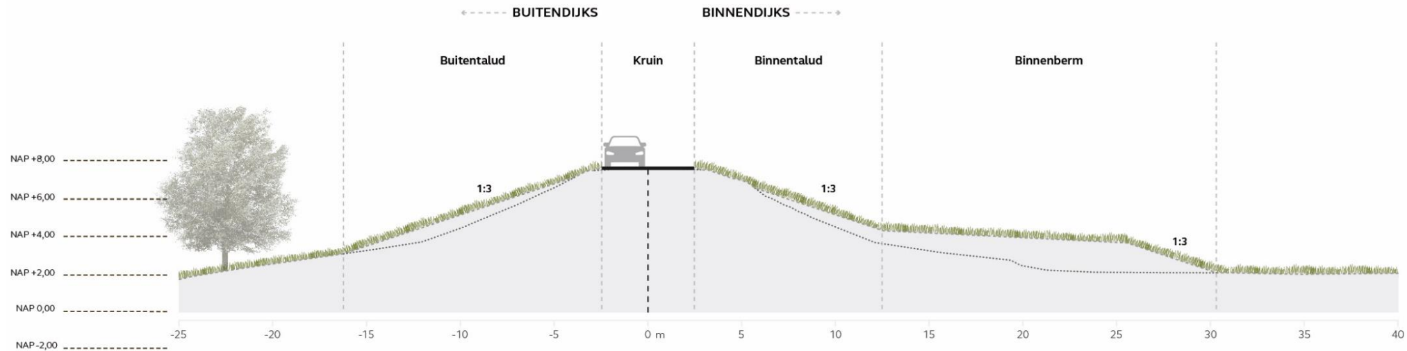
Dijkvak 25a Kruinverhoging en binnenberm (alternatief 1)
