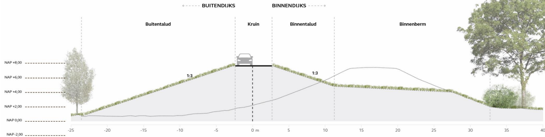
Dijkvak 26a Buitenwaartse asverschuiving (alternatief 2)
