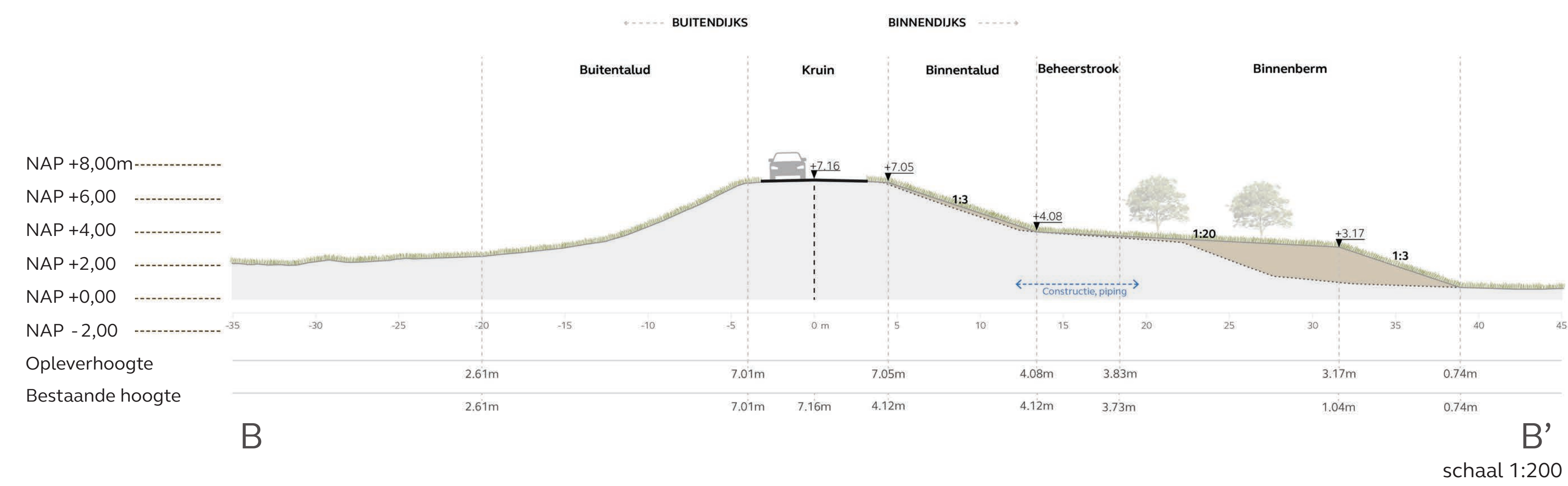
Profiel CC' Verbreding binnenberm
