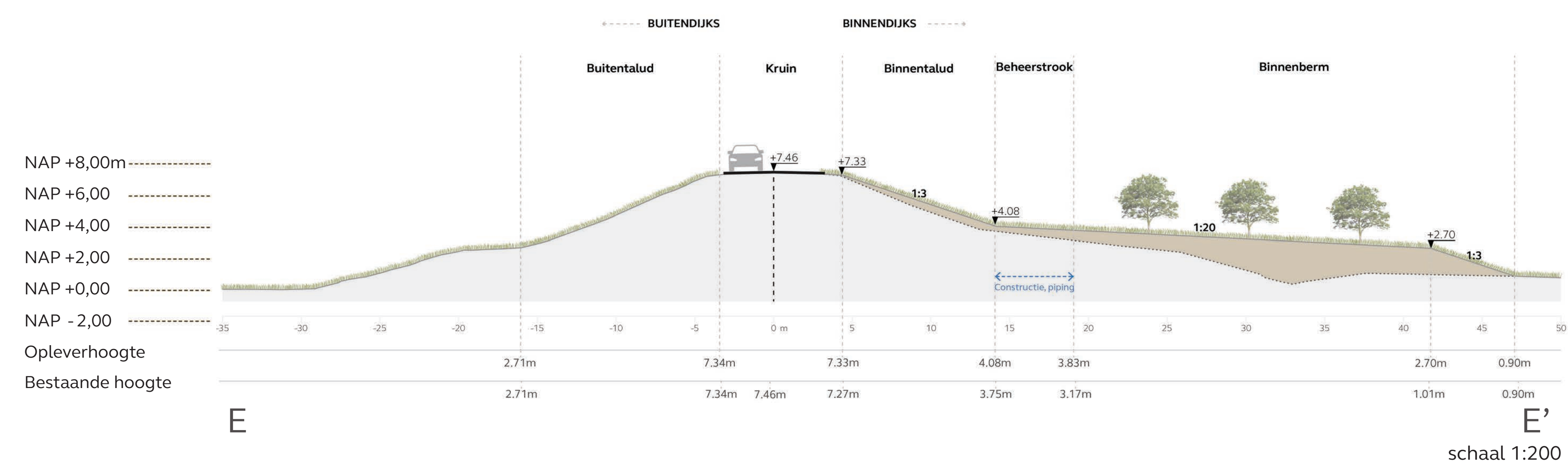
Profiel FF' Constructie stabiliteit en piping
