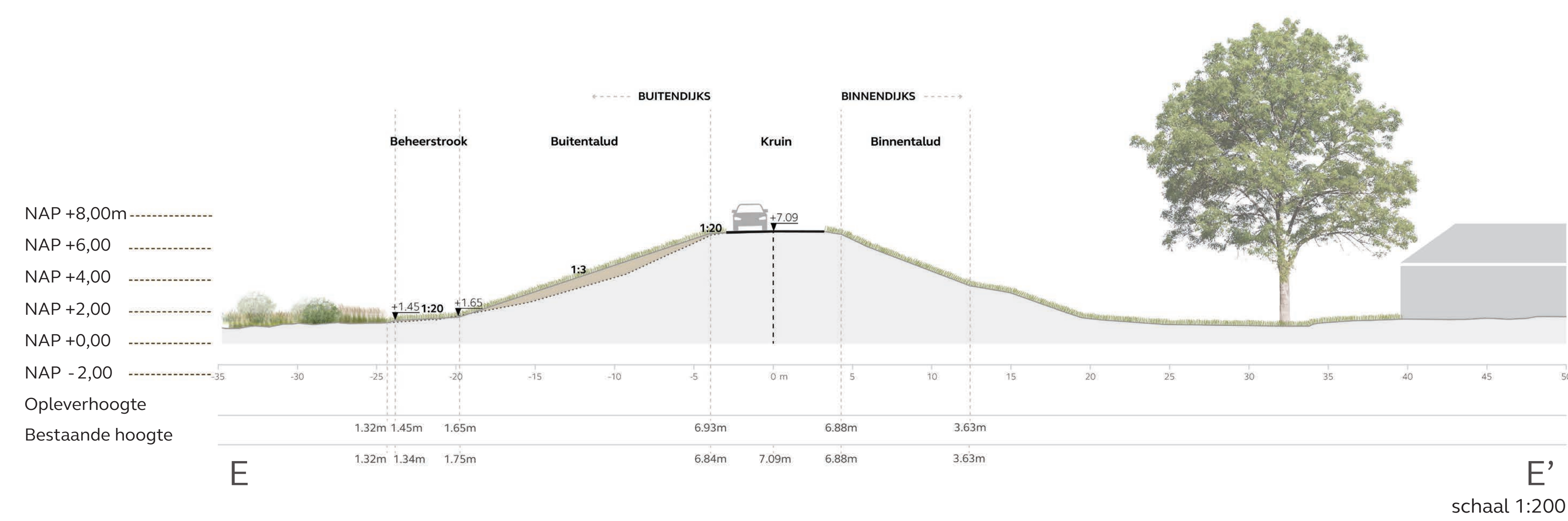
Profiel FF' Binnenberm en verflauwing buitentalud
