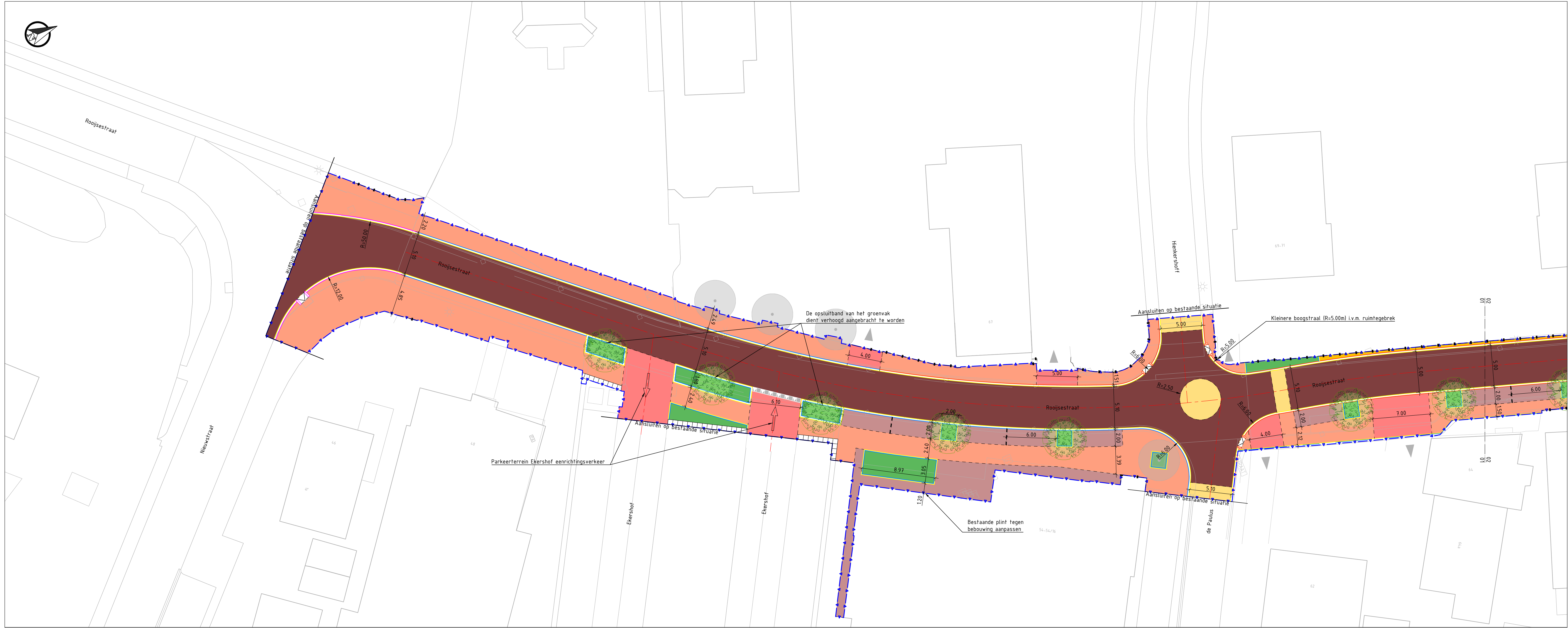
SITUATIE 051-1 SCHAAAL 1 : 200
