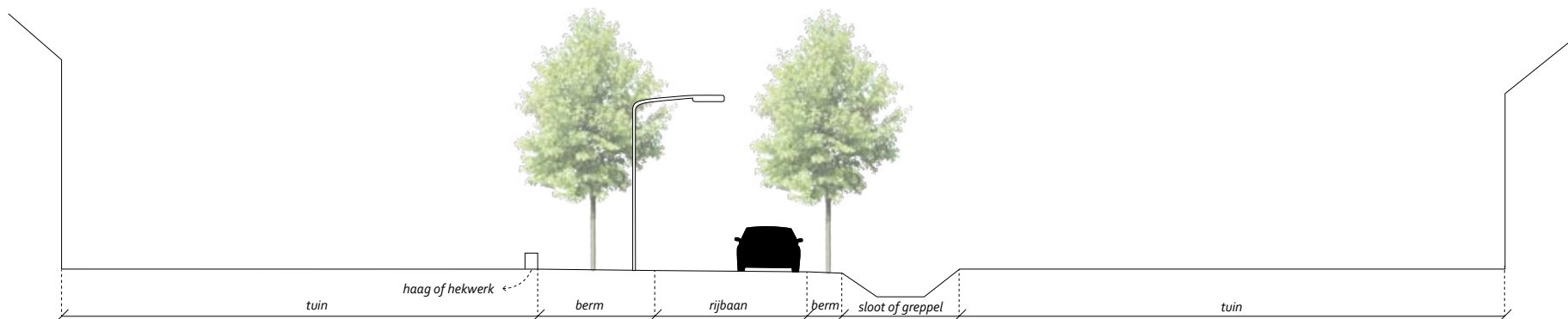
Basisprofiel landelijk lint
