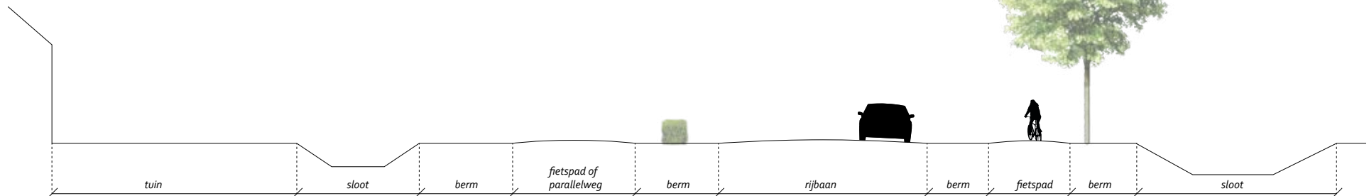
Basisprofiel Van Heemstraweg
