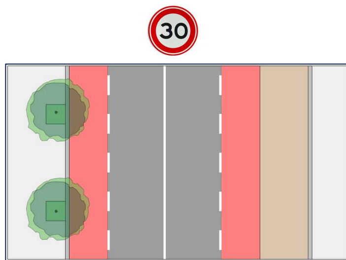
Figuur 7: Inrichting gebiedsontsluitingsweg 30
