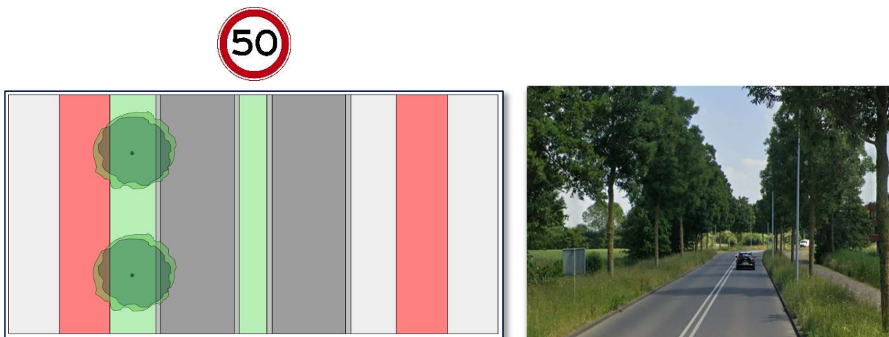
Figuur 5: Inrichting gebiedsontsluitingsweg 50 binnen de bebouwde kom
