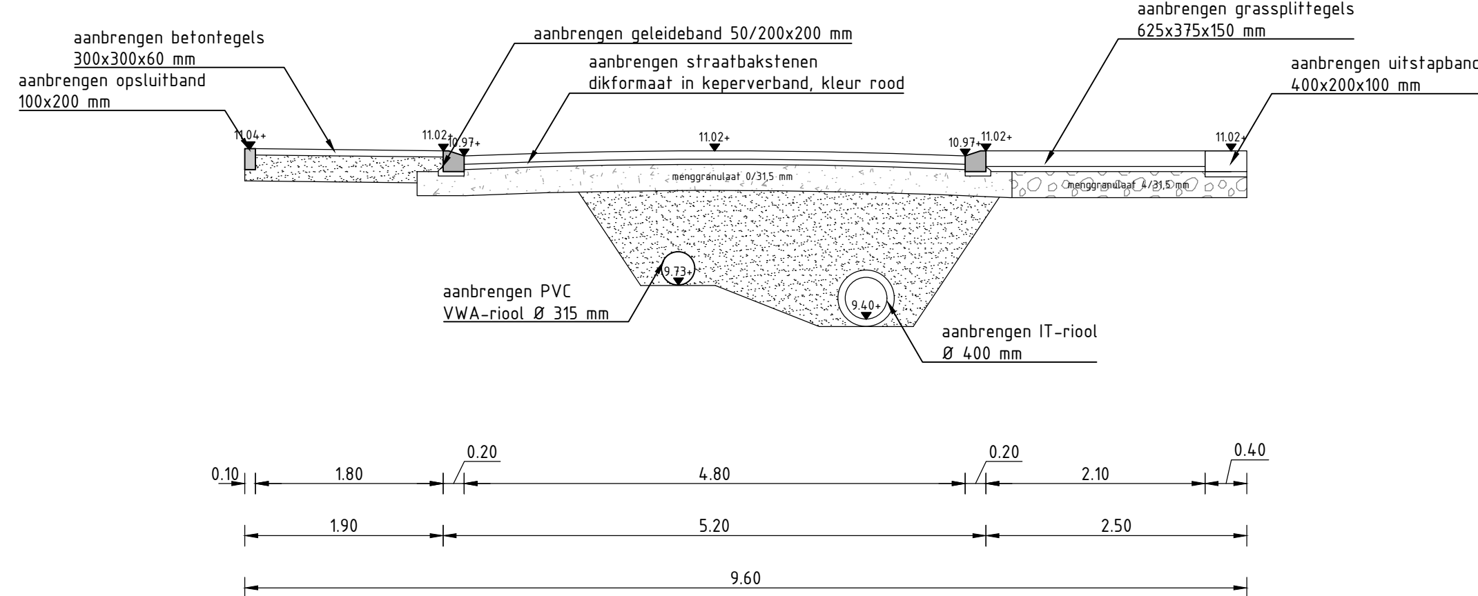
Doorsnede F-F
