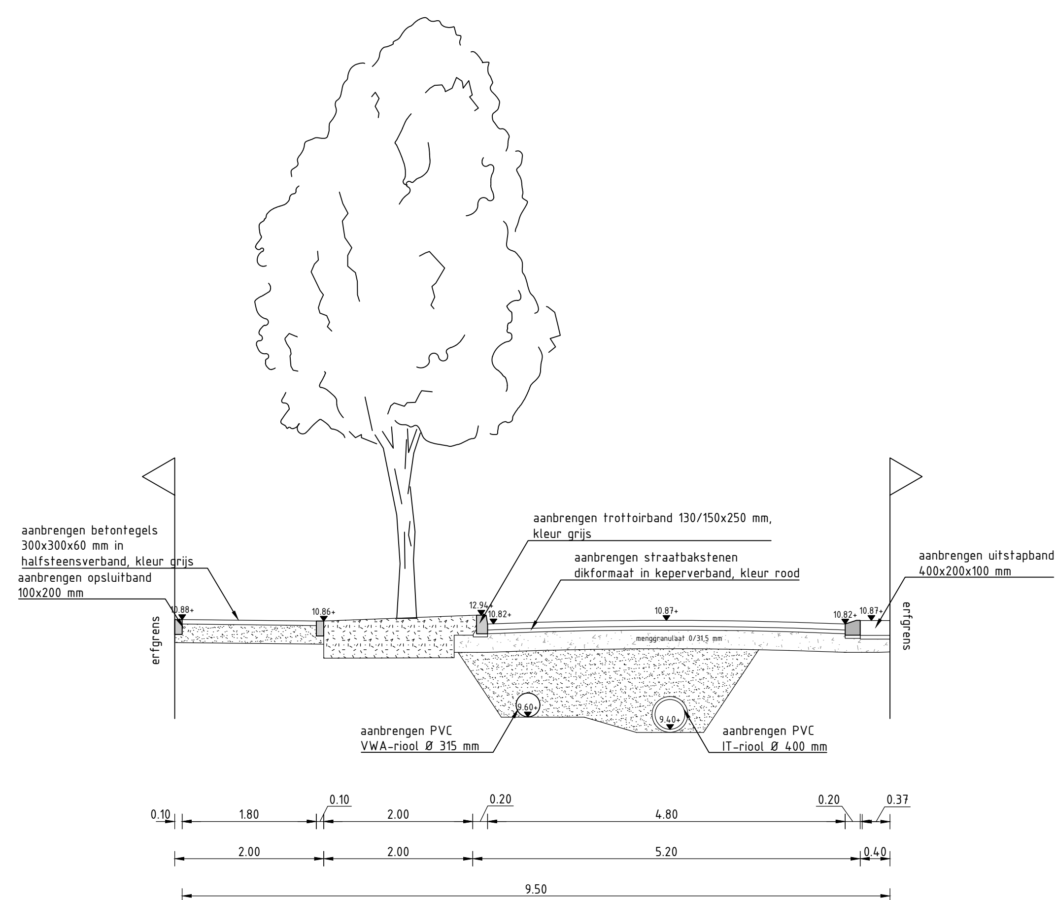
Doorsnede E-E
