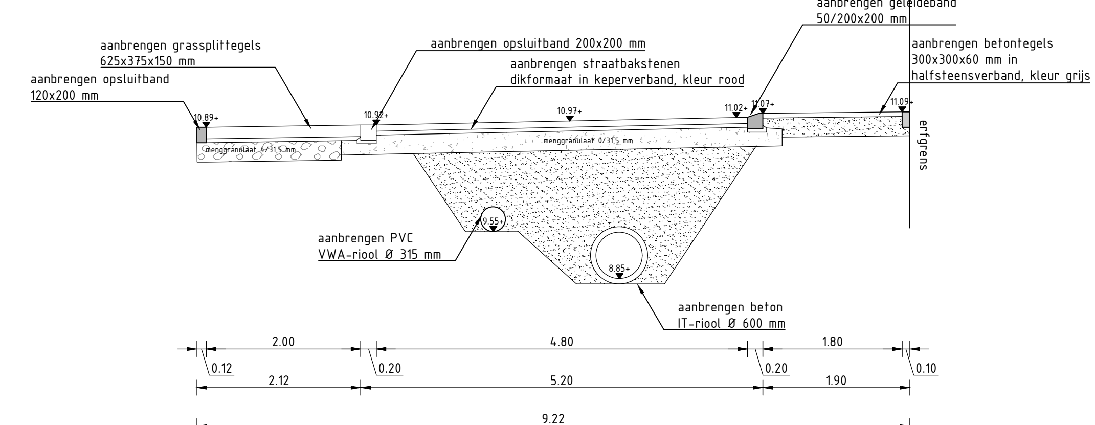
Doorsnede K-K
