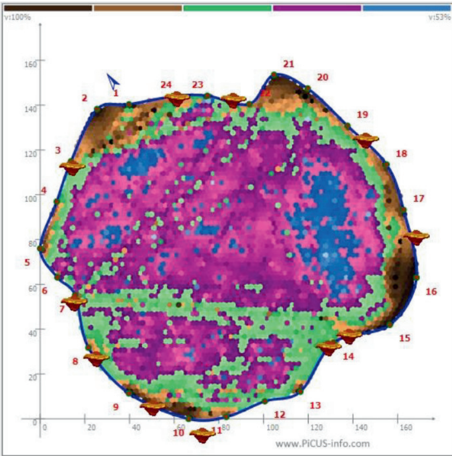
Om een beeld te krijgen van de houtkwaliteit in de stamvoet van de rode beuk is een geluidsmeting uitgevoerd op 50 cm boven maaiveld. De stamomtrek op 50 cm hoogte is 525 cm. De diameter is 167 cm. Op bovenstaande afbeelding is het tomogram te zien.
