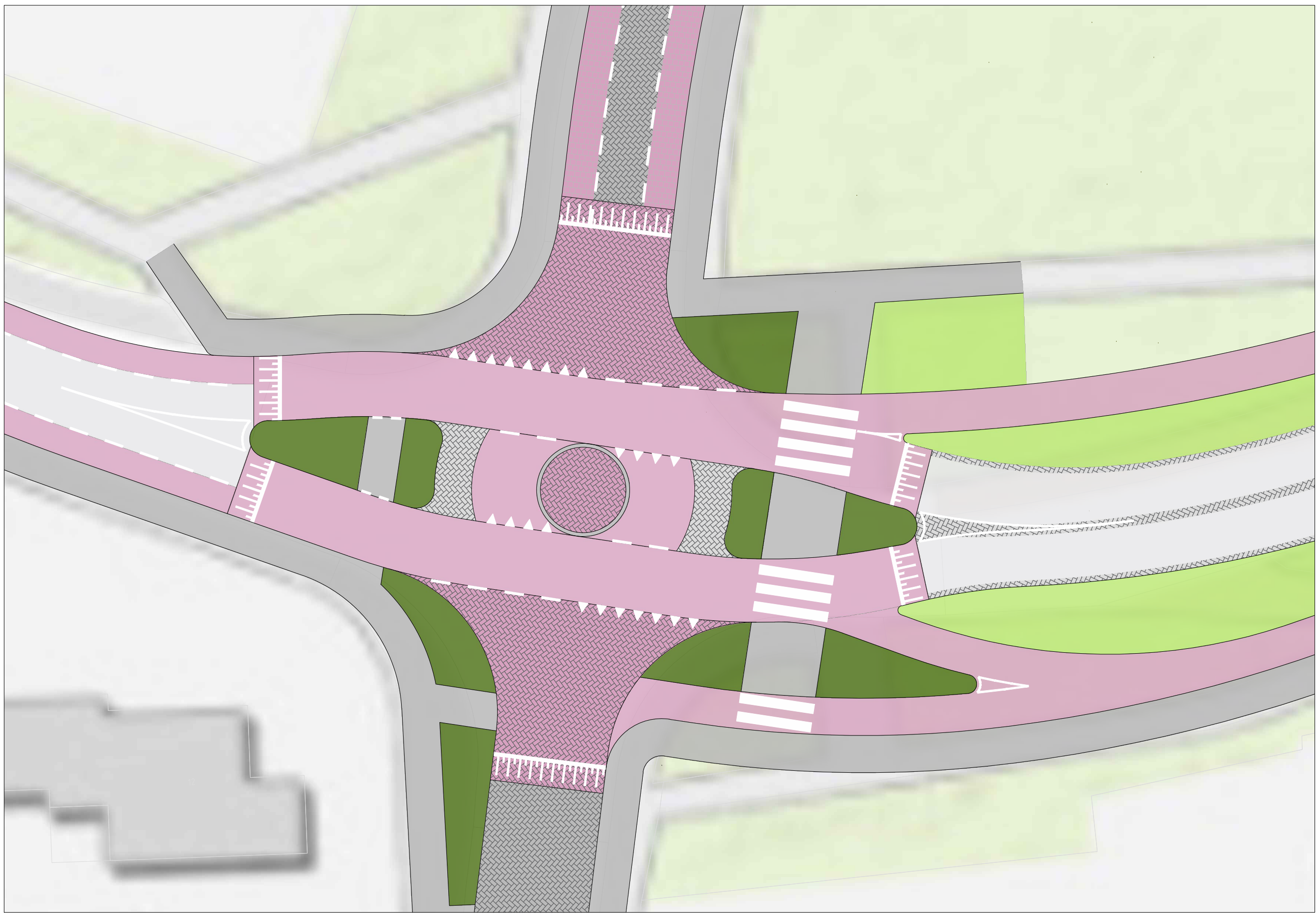
A - Detailtekening kruispunt Bornebroekseweg - Reggestraat (1:200)
