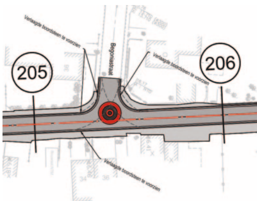
KRUISPUNT BEGONIASTRAAT • GRENSSTRAAT (NL)/ DRIEHOEVENSEWEG (BE)
