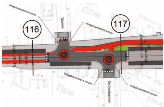
KRUISPUNT GRENSSTRAAT • TULPSTRAAT • ST. DIONYSIUSSTRAAT • DRIEHOEVENSEWEG (BE)
