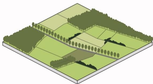
Oeverwallenlandschap (schematisch)
