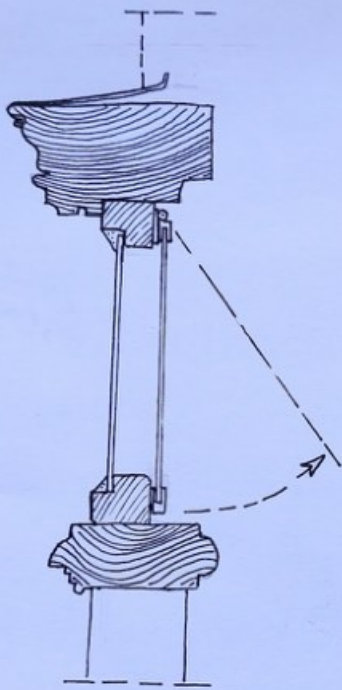
Doorsnede Bovenlicht
