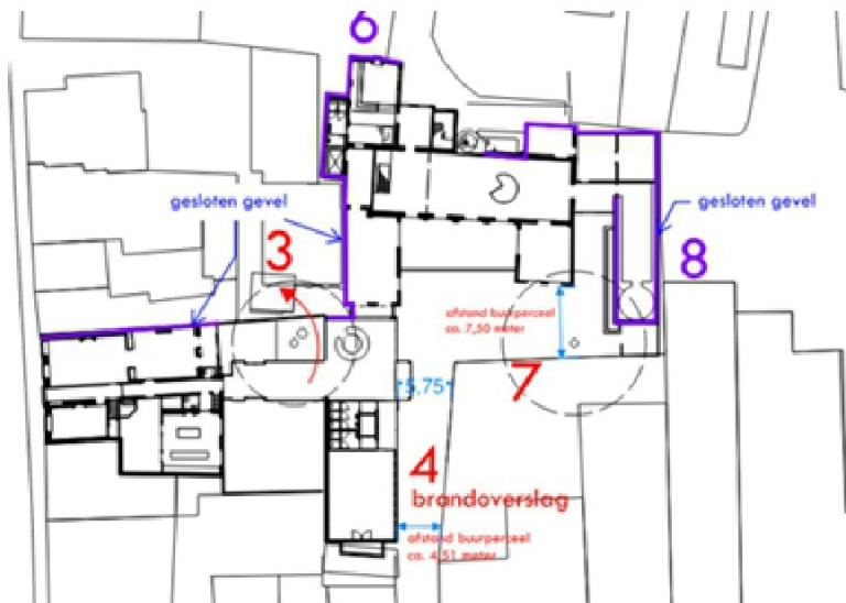
Figuur 6: brandoverslag situatie 6 en 8. De gevels grenzend aan buurpanden Gasthuisstraat en Herenstraat zijn gesloten uitgevoerd met een WBDBO 60 minuten, 60EI. Hier is geen risico op brandoverslag.
