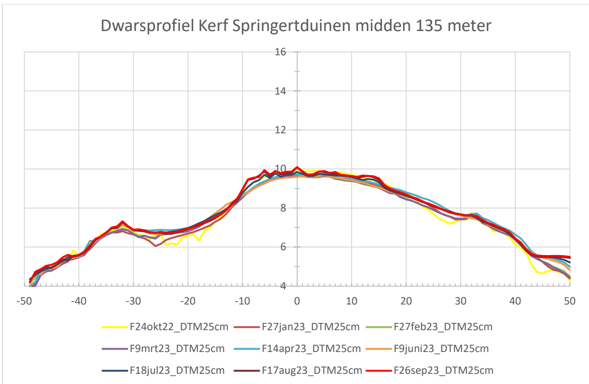
Figuur 11: Dwarsprofiel door middelste kerf, 135 m vanaf referentiepunt
