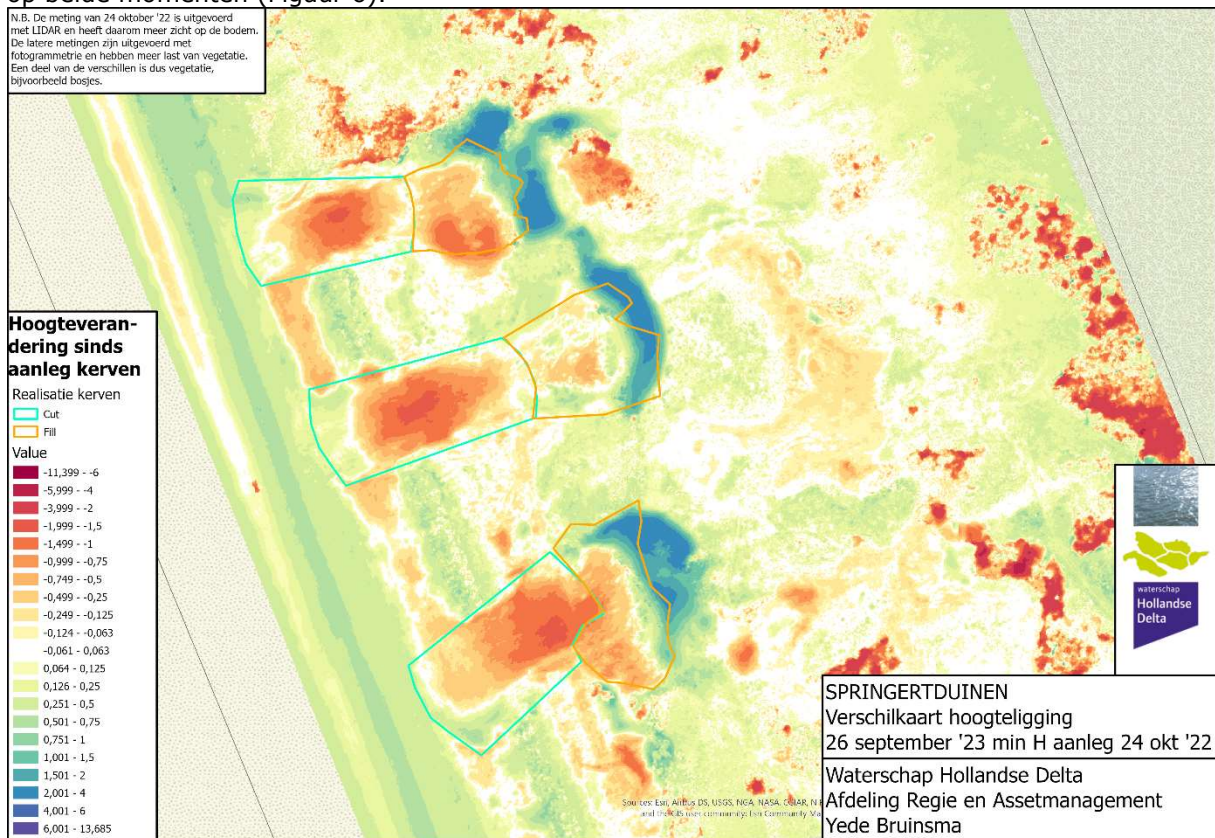
Figuur 6: Vershilkaart hoogteligging cluster 2 tussen 26 september 2023 en 24 oktober 2022
