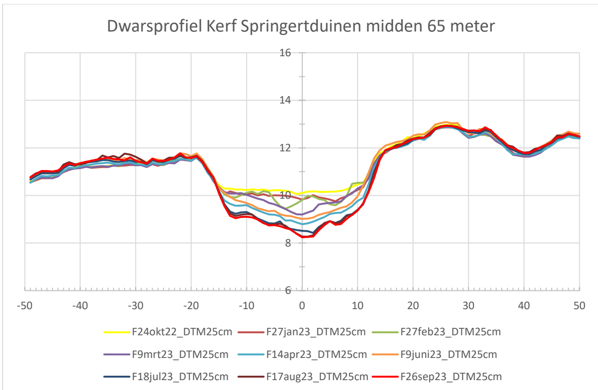
Figuur 9: Dwarsprofiel door middelste kerf, 65 m vanaf referentiepunt
