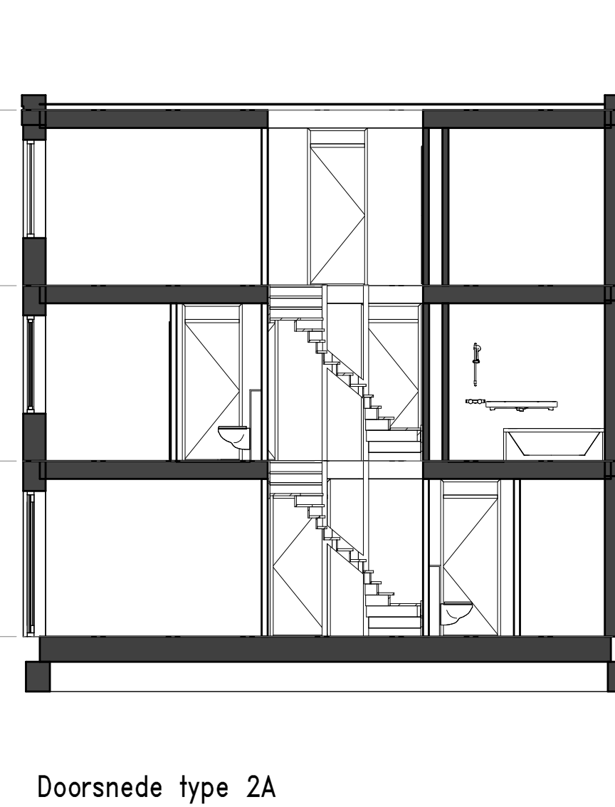
Doorsnede type 2A
