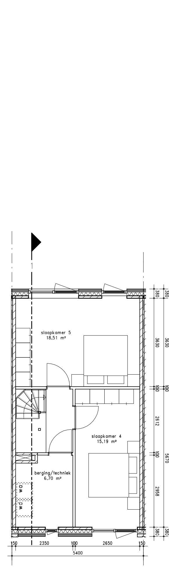
02 tweede verdieping Type 1
