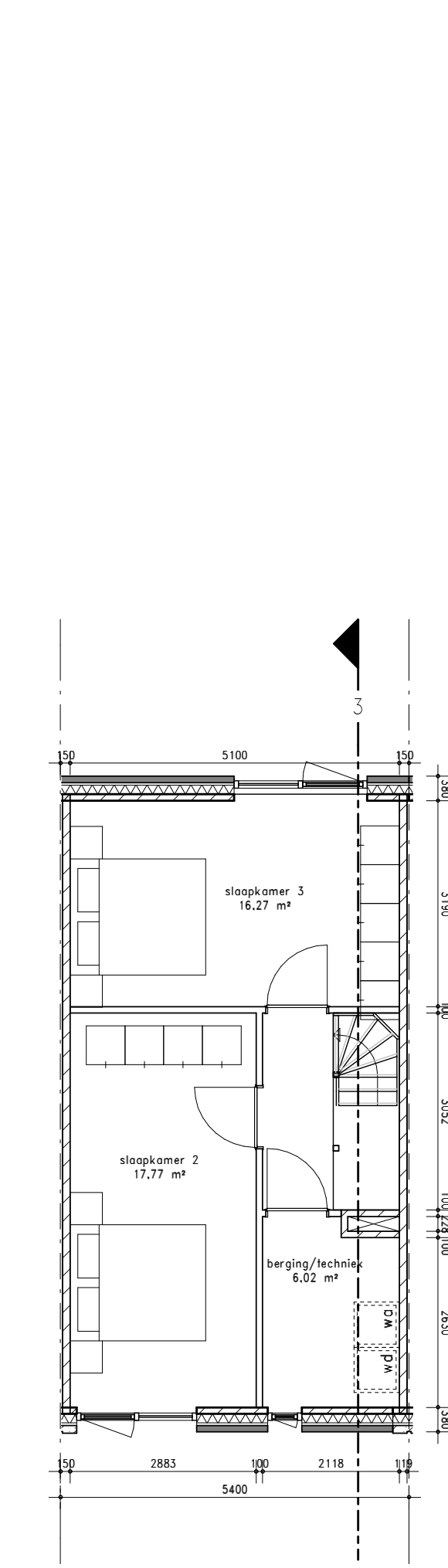
02 tweede verdieping Type 3
