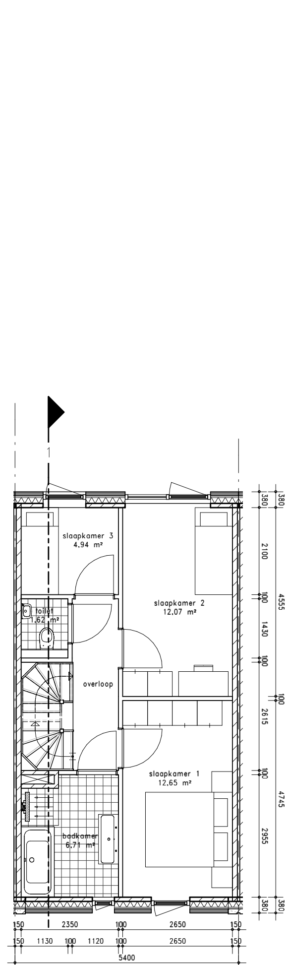
01 eerste verdieping Type 1
