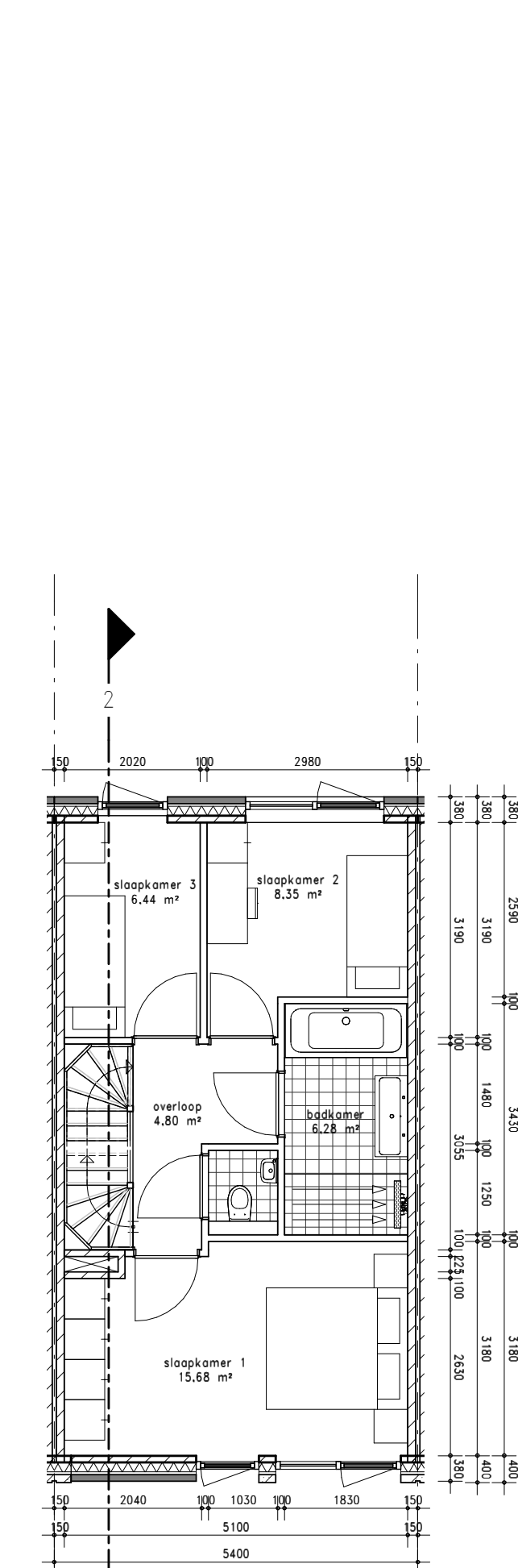
01 eerste verdieping Type 2
