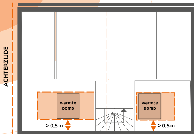
Geïntegreerde warmtepomp unit
