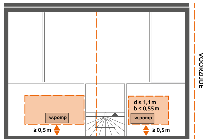
Warmtepomp unit in de vorm van een schoorsteen
