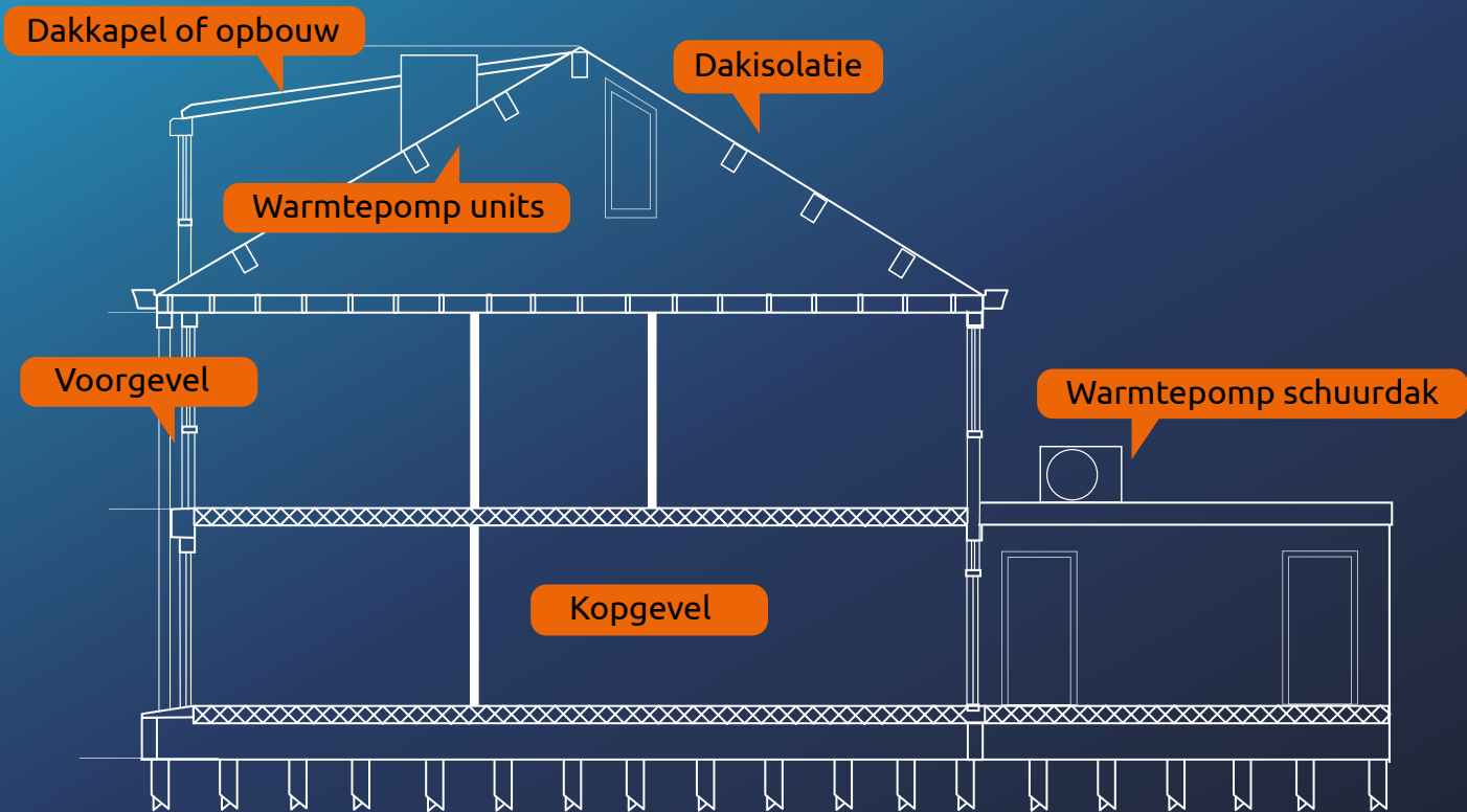
DOORSNEDE A-A
