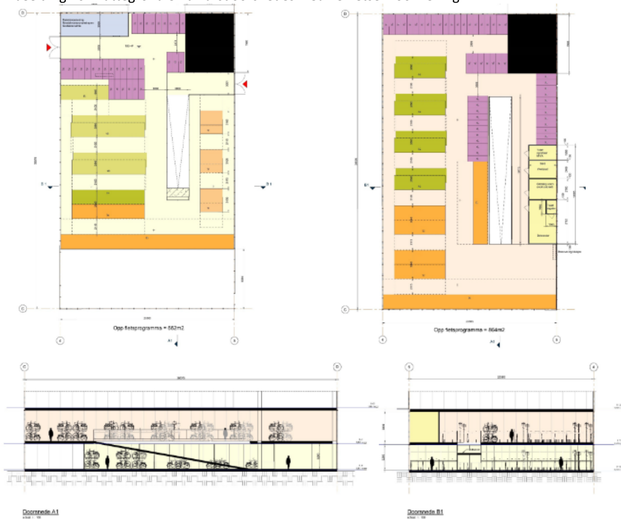
Afbeelding 10. Plattegrond en dwarsdoornedes nieuwe fietsenvoorziening
