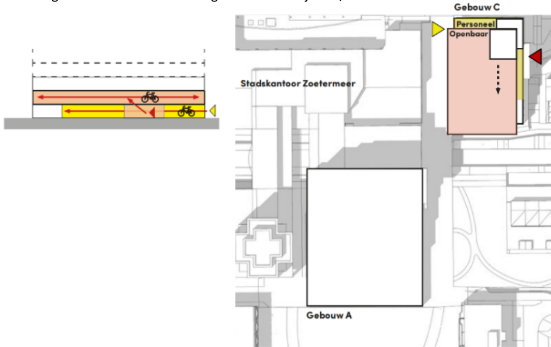
Afbeelding 9. Nieuwe fietsvoorziening locatie Frankrijklaan/ Reimsstraat
