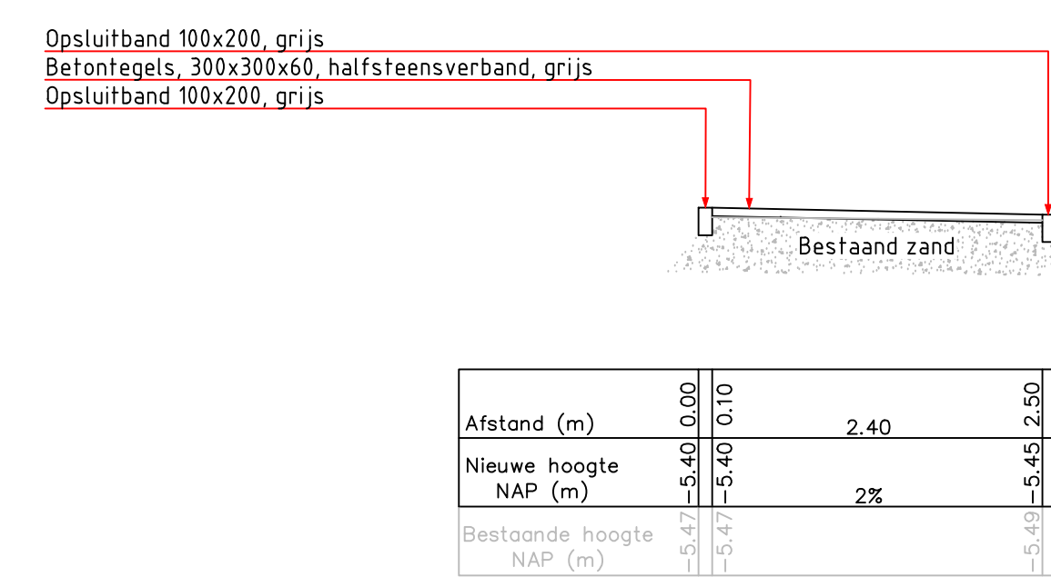
DWARSDOORSNEDE A-A' Nieuwe situatie Schaal 1:50
