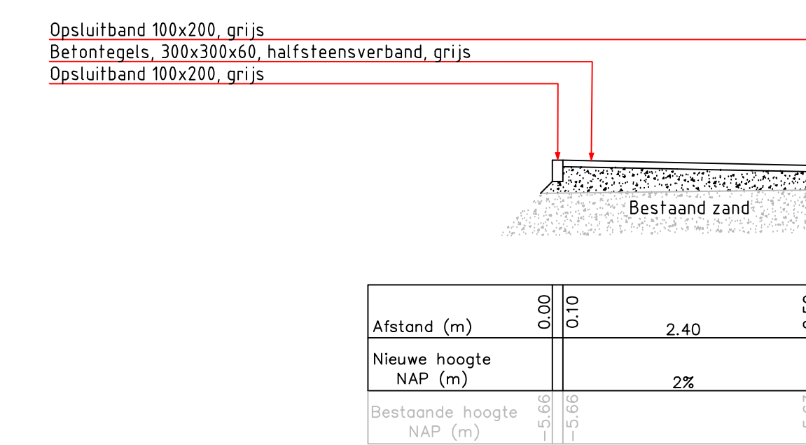
DWARSDOORSNEDE C-C' Nieuwe situatie Schaal 1:50
