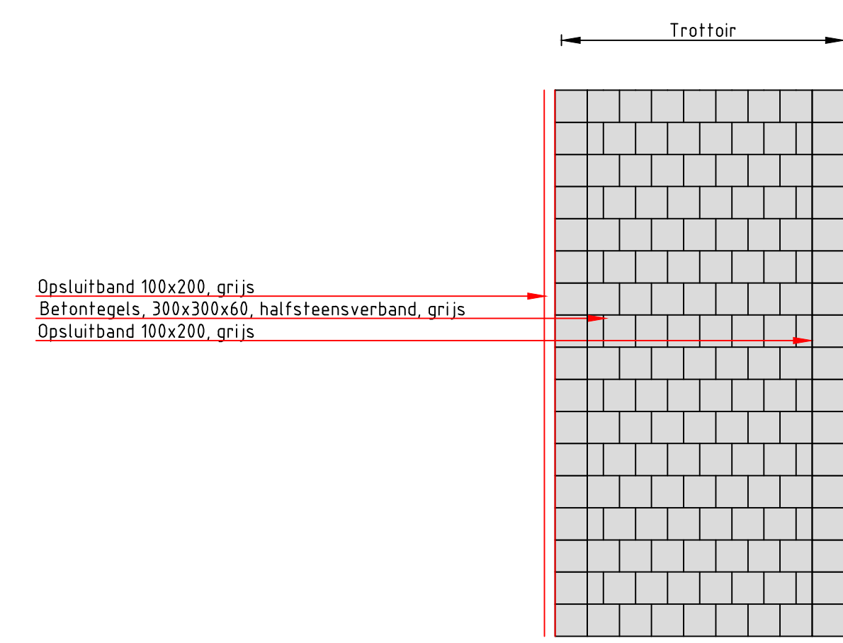
PRINCIPE DETAIL B-B' Nieuwe situatie Schaal 1:50
