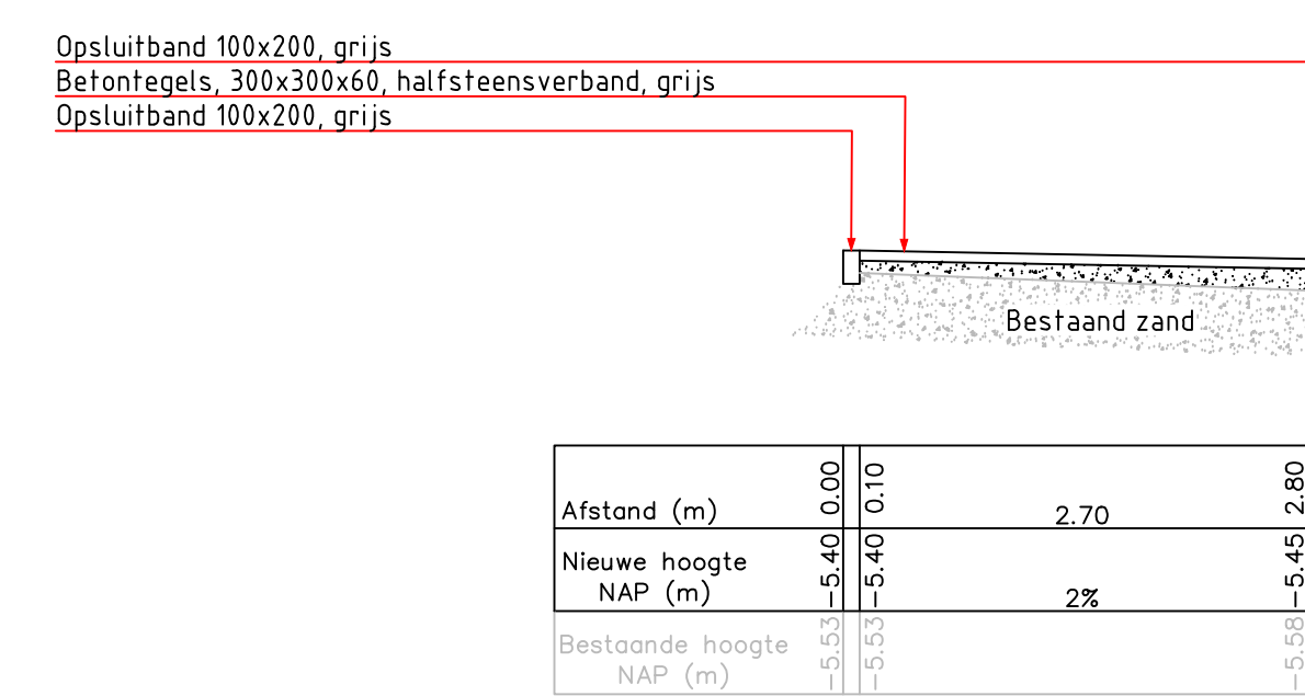
DWARSDOORSNEDE B-B' Nieuwe situatie Schaal 1:50
