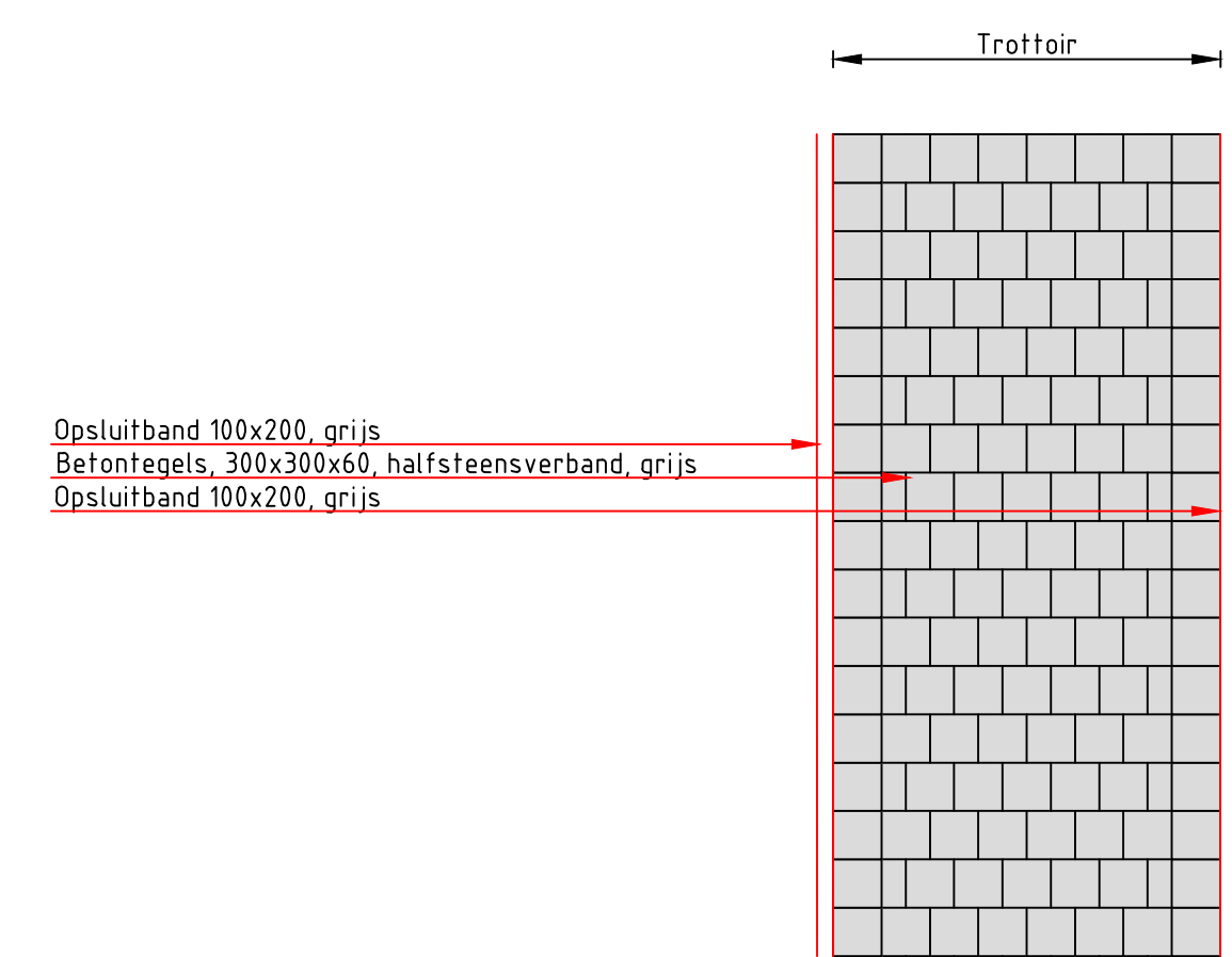
PRINCIPE DETAIL E-E' Nieuwe situatie Schaal 1:50
