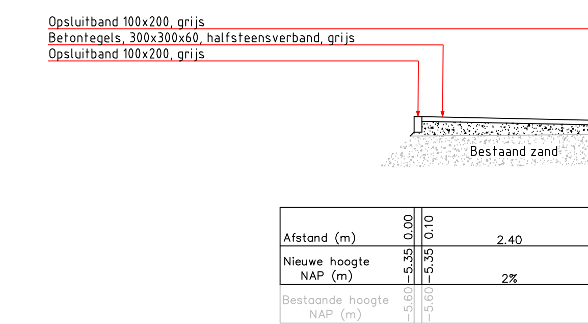
DWARSDOORSNEDE D-D' Nieuwe situatie Schaal 1:50
