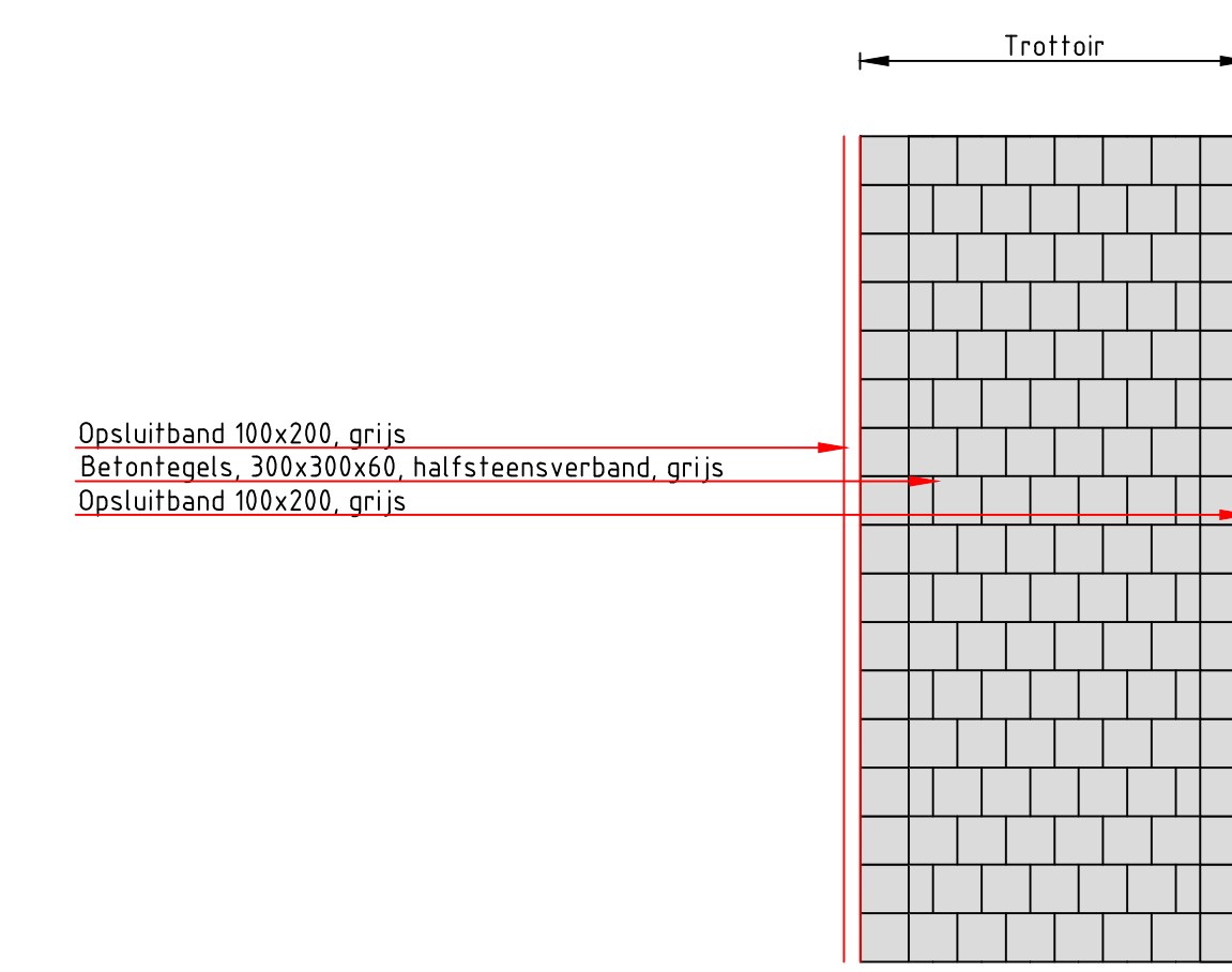
PRINCIPE DETAIL C-C' Nieuwe situatie Schaal 1:50
