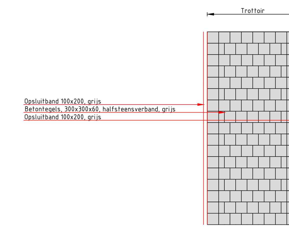
PRINCIPE DETAIL D-D' Nieuwe situatie Schaal 1:50
