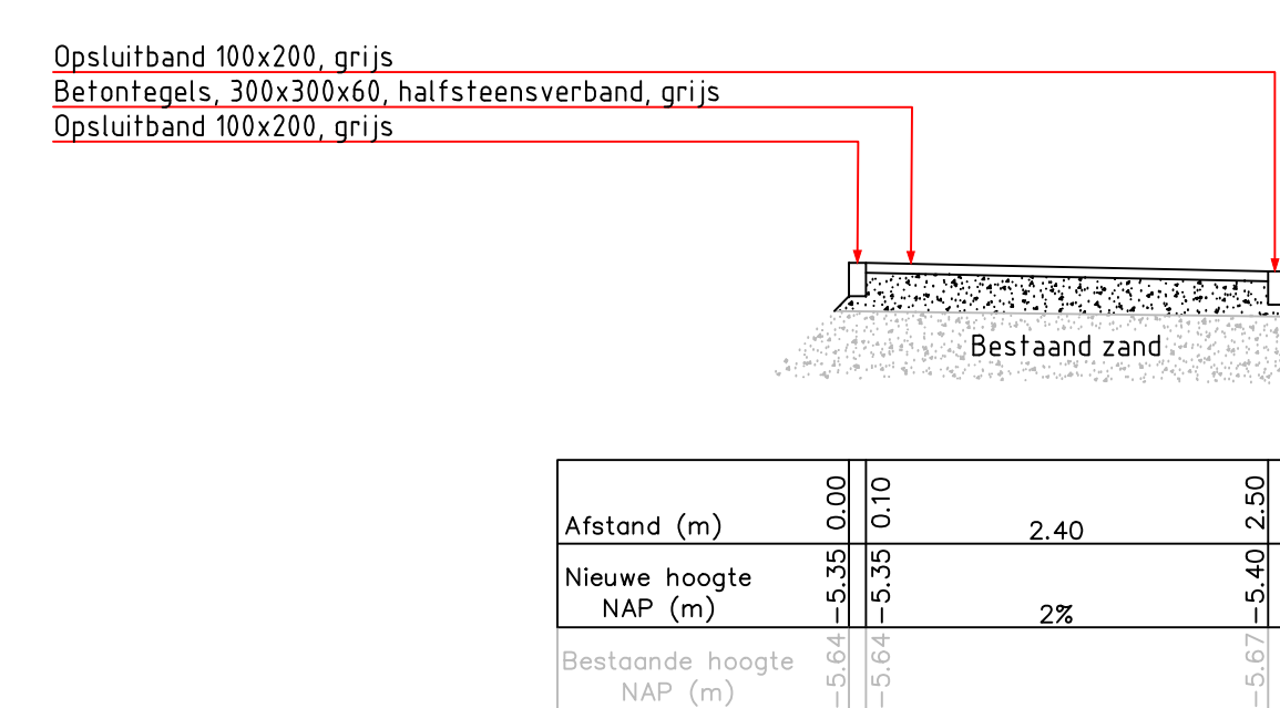
DWARSDOORSNEDE E-E' Nieuwe situatie Schaal 1:50
