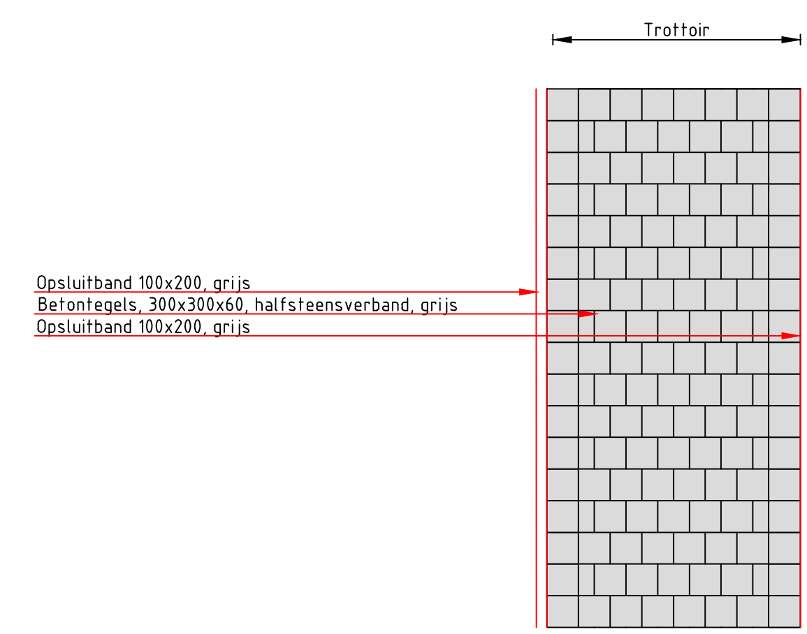
PRINCIPE DETAIL A-A' Nieuwe situatie Schaal 1:50
