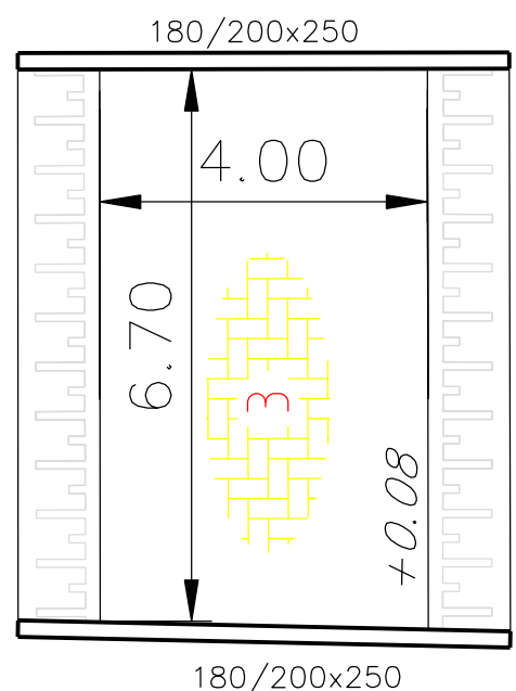
detail 1 schaal1:100
