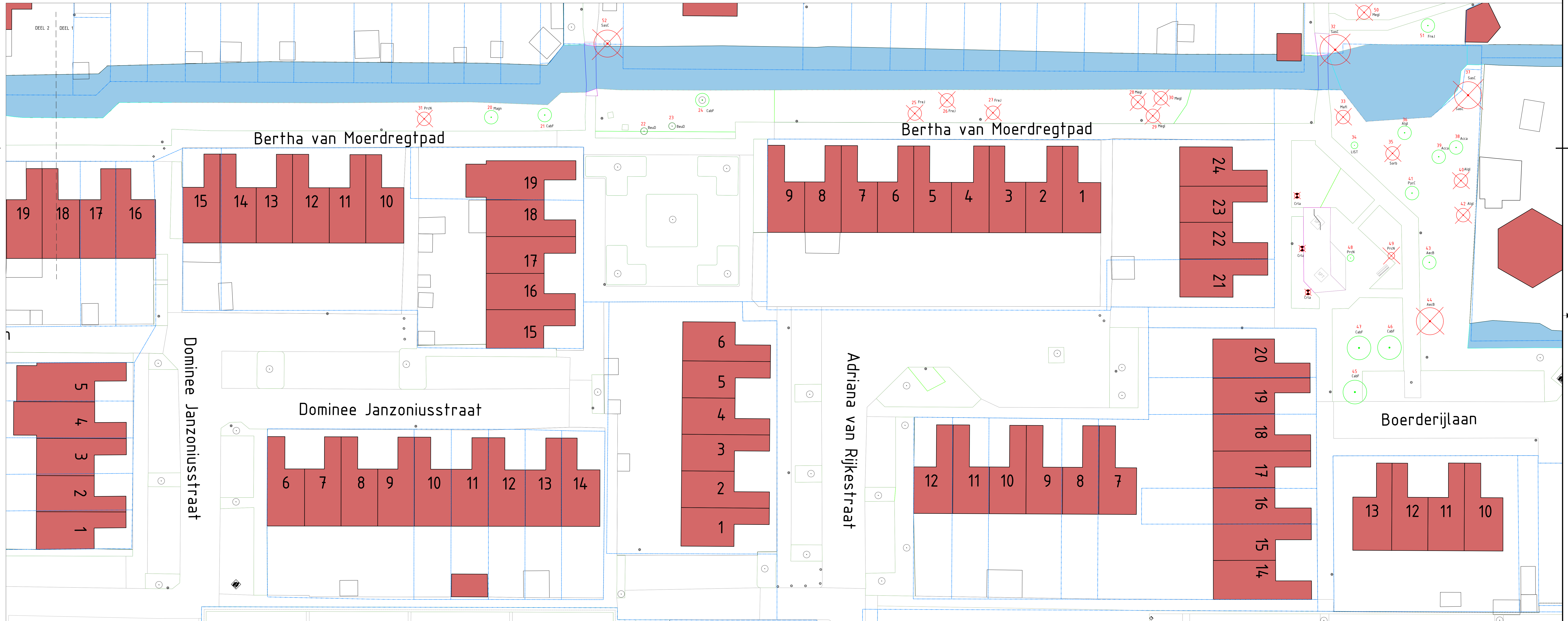
Bovenaanzicht Moerdregtpad deel 1 SCHAAL 1 : 200
