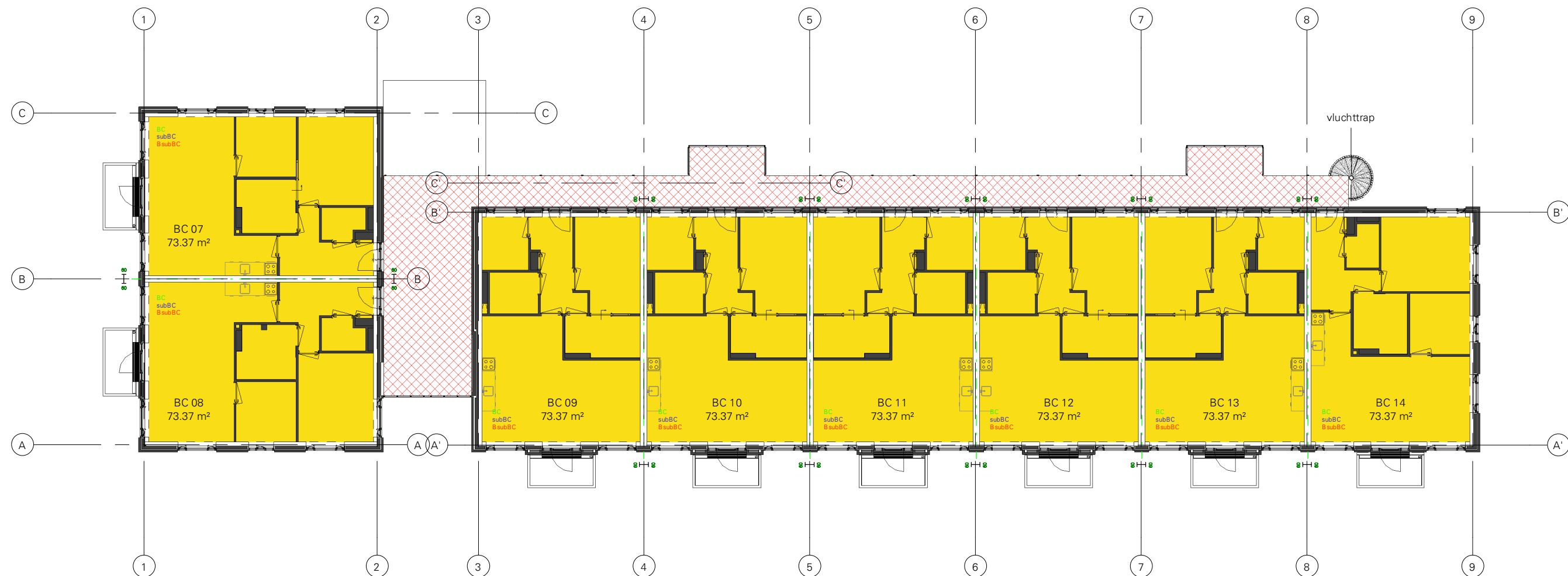
01 eerste verdieping
