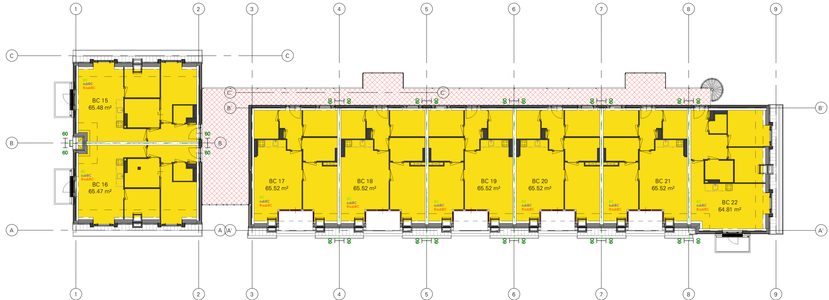
02 tweede verdieping
